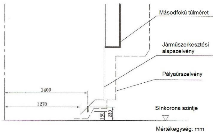
5.b ábra Az 1435 mm-es nyomtávolságú vasutak raxszelvénye: KZD (másodfokú alsó túlméret)
